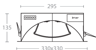
Découpe plafond 315x315
